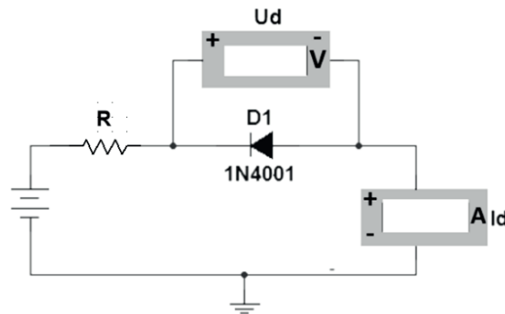
Slika 3. Shema spoja za zapornu polarizaciju energetske diode Figure 3 Diagram for reverse biasing of a power diode
